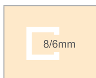
Üveg Ajtó 8mm Rögzített szegmens 6mm
