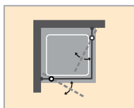
Sarokbelépő nyílóajtó fix részel
